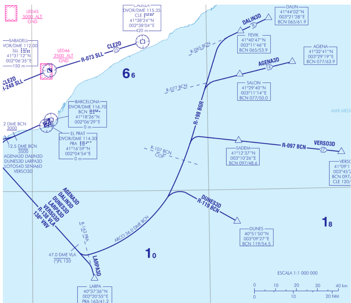
Figura 3.21: Extracto de SID convencional de la RWY 25R de LEBL [Fig27].
